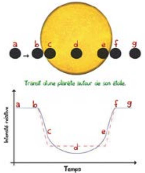
Transit d'une exoplanète : en passant devant son étoile, la planète fait baisser légèrement sa lumière. Les astronomes le voient sur la courbe de luminosité au fil du temps, comme ici ci-dessus.
