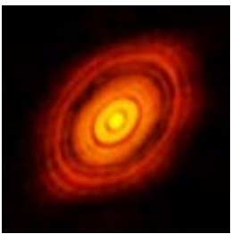
< HL Tauri, disque protoplanétaire avec ses planètes en formation, à moins de 100000 ans. Photographié en 2014.
